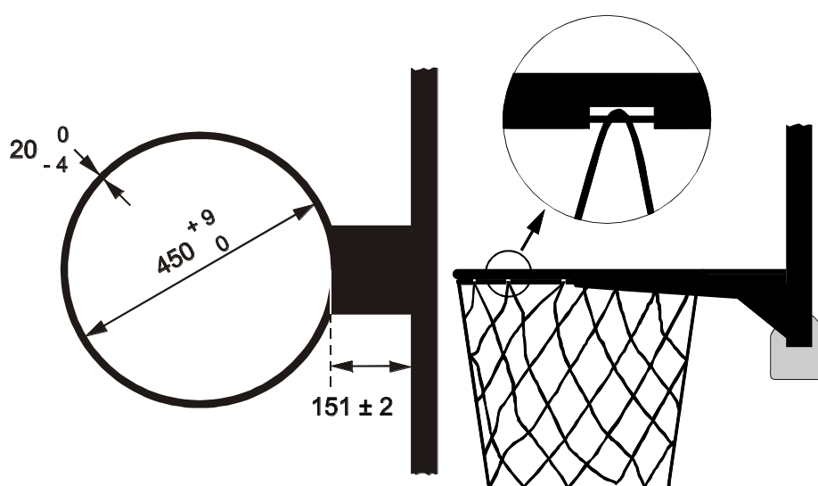
Netzbefestigung (Beispiel)
